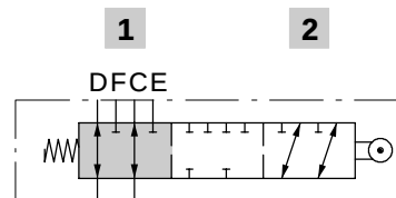
Spool type B
