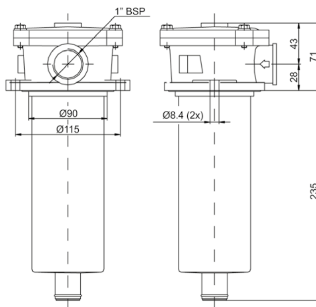
3 Filtro para depósitos/ Oil filter for tanks 140 L., 160 L., 200 L. Código Part Number: 901410
