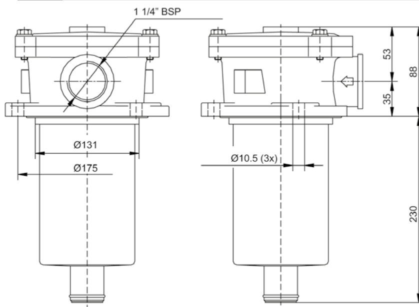
3 Filtro para depósitos/ Oil filter for tanks 140 L., 160 L., 200 L. Código Part Number: 901410
