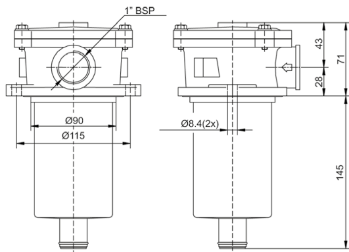
1 Filtro para depósitos/ Oil filter for tanks 30 L. , 60 L. Código Part Number: 901510
