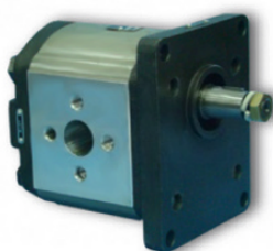
7 wałek stożkowy 1:8
