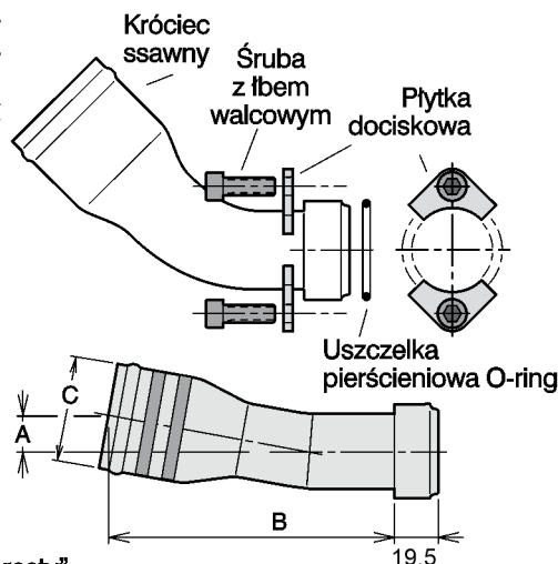
Króciec „prosty”
