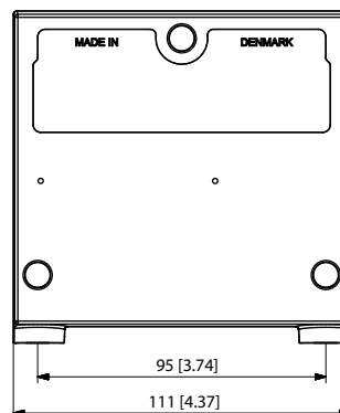
PVSI dimensions
