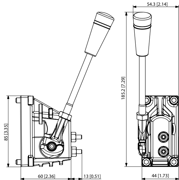
PVM dimensions
