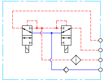
PVEO/PVEO-DI schematic
