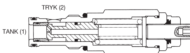
Direkte styret ventil
