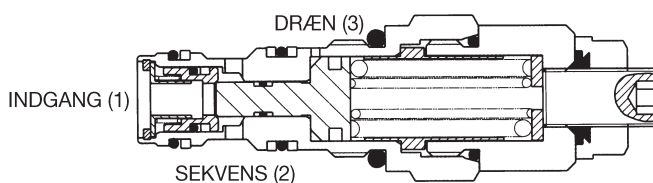
Sekvensventil med kontraventil
