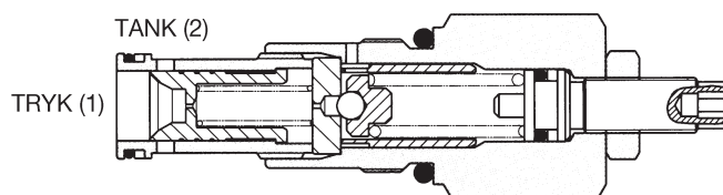
Pilotstyret ventil
