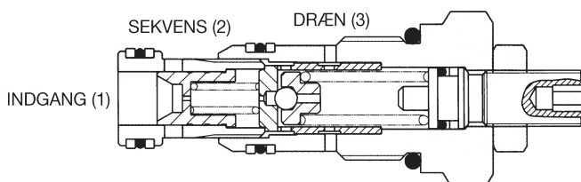
Sekvensventil uden kontraventil
