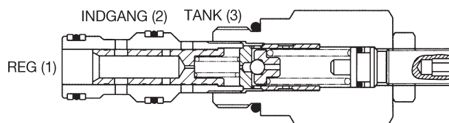
Reduktionsventil med aflastning
