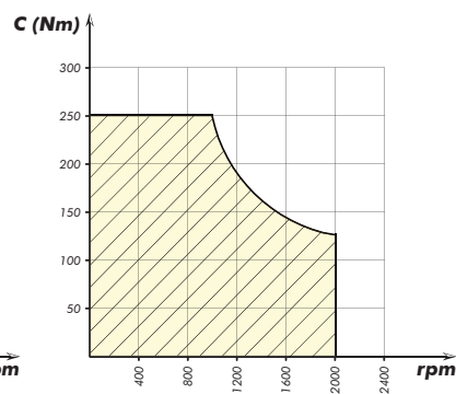
Diagramma di utilizzo Working conditions
