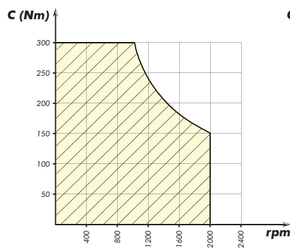
Diagramma di utilizzo Working conditions
